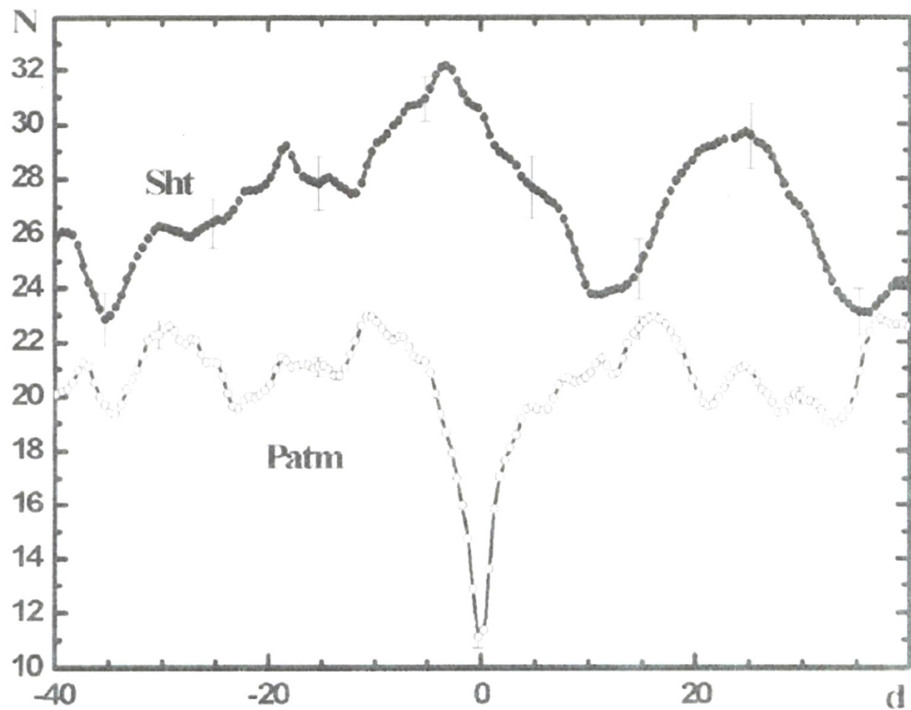
Рис. 6 Средний профиль интенсивности кристаллообразования относительно суток, в которых барометрическое давление либо сильно падало, либо возрастало. График построен методом наложения эпох (пояснение в тексте).
