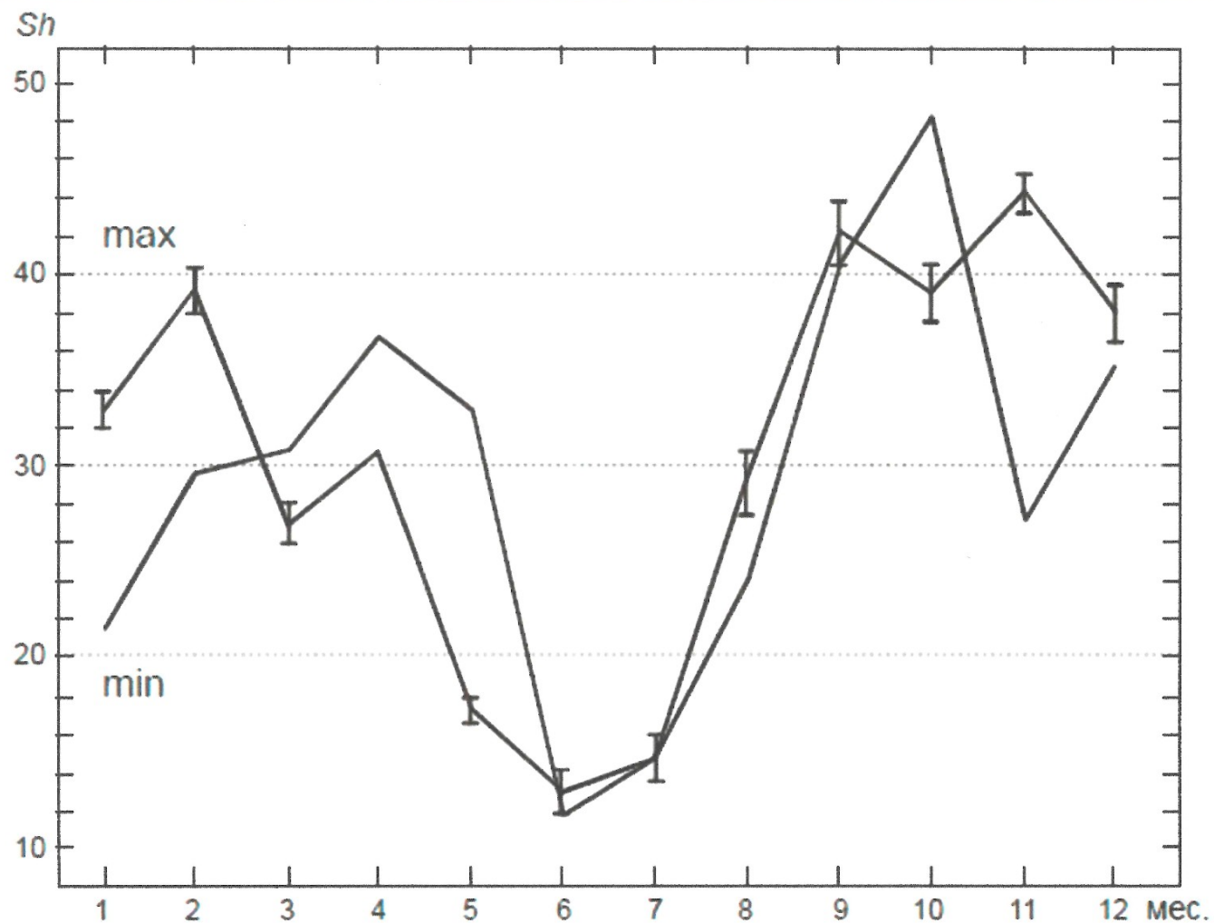
Рис. 1. Годовой ход усредненных по нескольким приборам среднемесячных значений интенсивности кристаллизации Sh (мм) в колбе Фицроя – штормглассе в 1996–2015 гг. отдельно для эпох максимума (max) и минимума (min) солнечной активности
